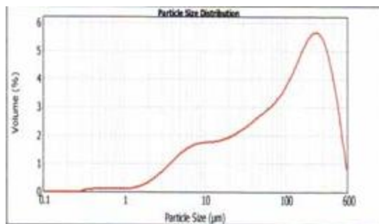
Fig.3c. Granulometrie cu laser-zgura de termocentrala
