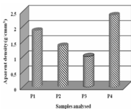
Fig.4a. Densitatea aparenta pentru probele analizate
